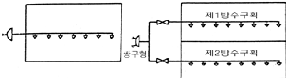
[그림 1-104] 연결살수설비 계통도
